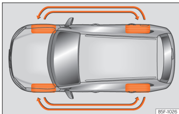
SL. 181 Premještanje kotača
