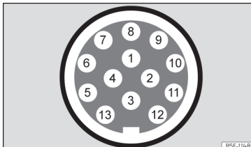
Sl. 142 Shematski prikaz: raspored zatika utičnih spojeva za struju prikolice.
