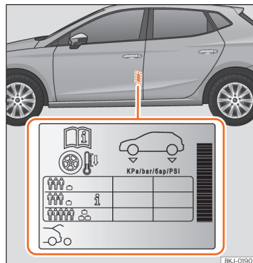
Sl. 179 Mjesto ugradnje naljepnice za tlak u gumama.
