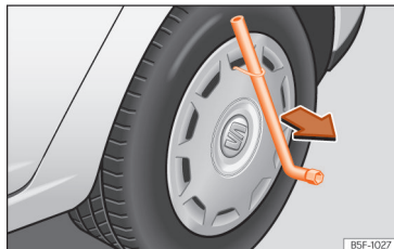
Sl. 184 Skidanje ukrasnog poklopa s kotača.
