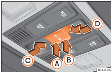
Sl. 60 U krovnoj oblozi: element za rukovanje za panoramski pomični krov.
