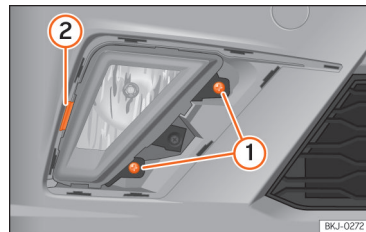
Sl. 164 Svjetla za maglu: demontaža nosača žaruljice
