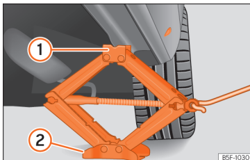
SL. 190 Uzdužni nosač: postavljanje dizalice vozila.
